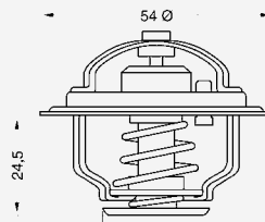
Typ 4003 ohne Entlüftungsventil oder -kerbe 4008 mit Entlüftungsventil 4015 mit Entlüftungsventil
