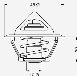
Typ 3017 3091 mit Entlüftungskerbe mit Entlüftungsventil und gummibeschichteter Ventilplatte 3082 gummibeschichtete Ventilplatte
